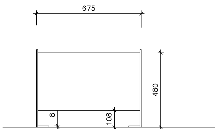
VY - PLANTERINGSKÄRL 2
