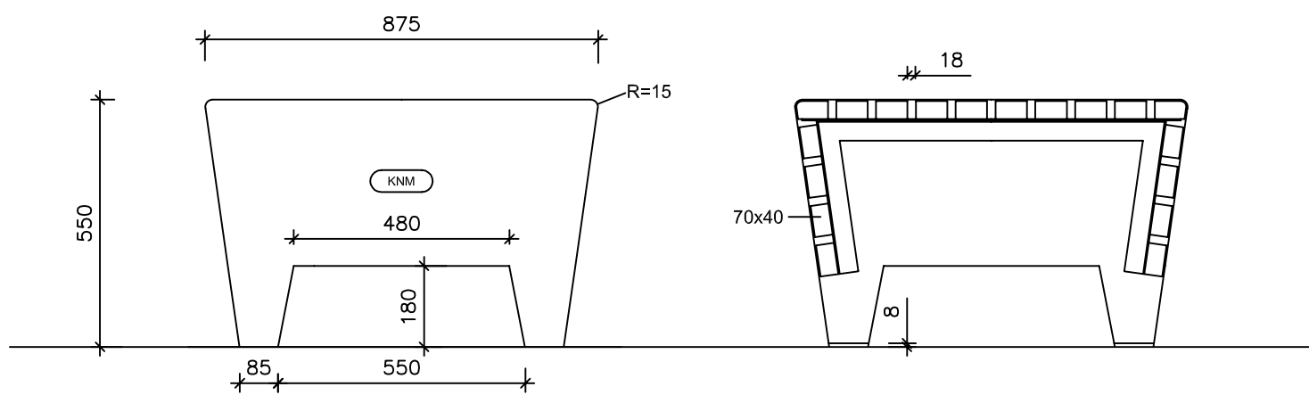
SEKTION - BÄNK
