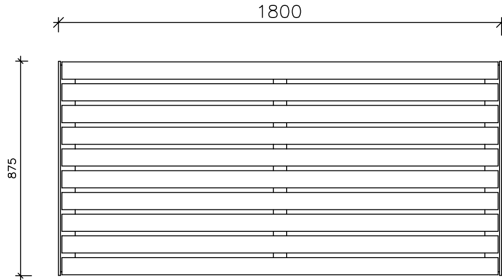
PLAN - BÄNK
